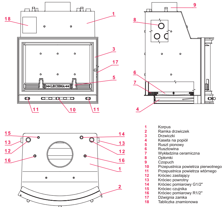
rys.3 Schemat budowy wkładu kominkowego z zespołem wodnym typu LECHMA PL-190 PANORAMA
