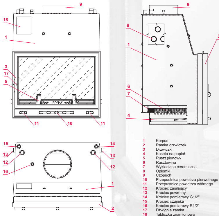
rys.1 Schemat budowy wkładu kominkowego z zespołem wodnym typu LECHMA PL-190
